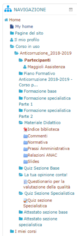
Figura 3 – menù
